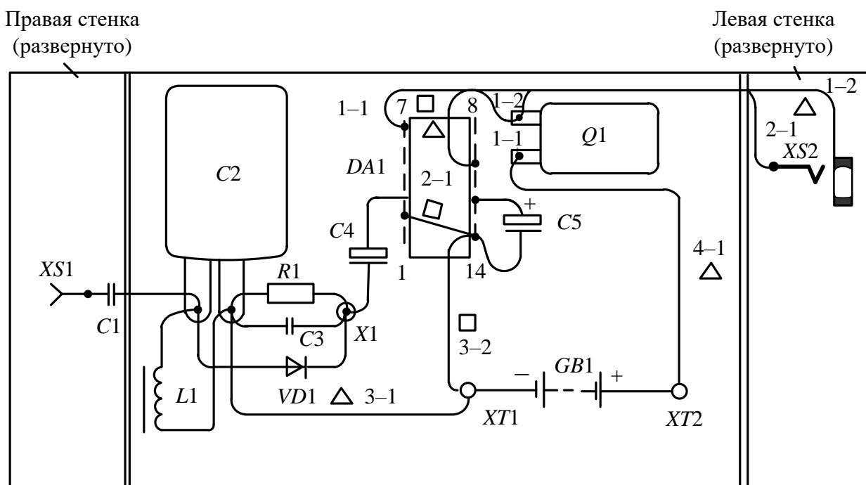
Рисунок 3.34 – Пример выполнения схемы соединений (Э4)
