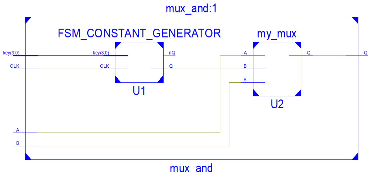
Рисунок 2 – Функционально эквивалентное описание простого логического элемента AND2 с использованием генератора константных значений и мультиплексора
