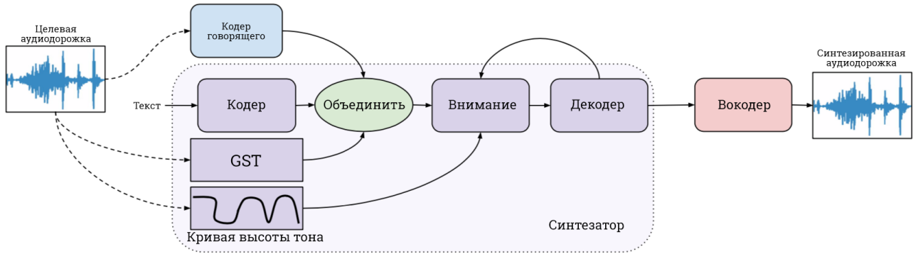
Рисунок 1 – Модель клонирования голоса Tacotron-2 TTS
