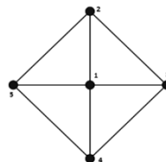
Рисунок 3 – граф-колесо порядка 3
